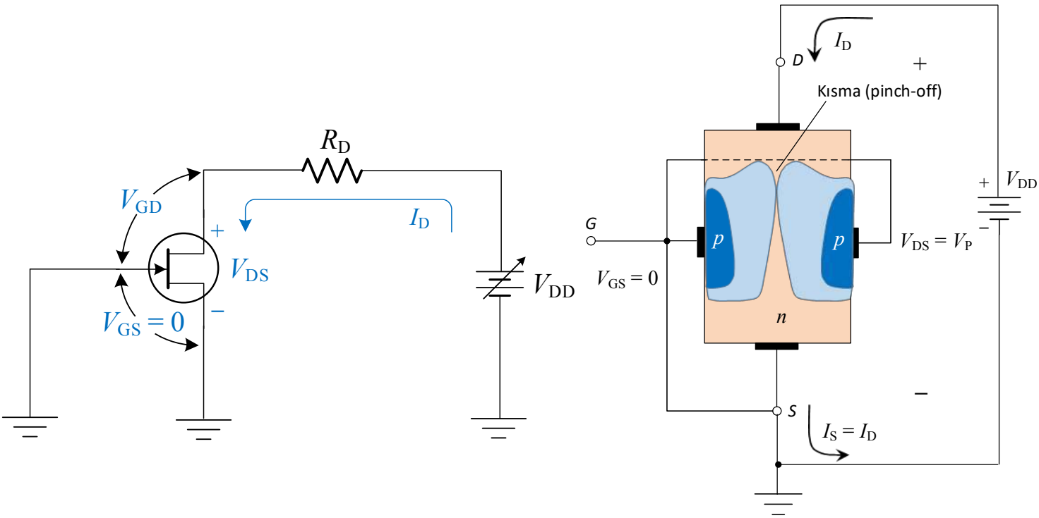
Şekil 4 a) V_{GS} = 0 ve değiştirilebilir V_{DS} ( V_{DD} ) ile JFET
