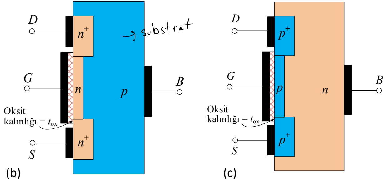
Şekil 13 n -kanal (NMOS) D-MOSFET'in fiziksel yapısı. (a) Derinlikli görünüm. (b) Kesit görünüm. (c) p -kanal. Tipik olarak L = 1.3 \mu\text{m} ile 1 \mu\text{m} aralığı, W = 0.1 \mu\text{m} ile 100 \mu\text{m} aralığına sahiptir. Oksit tabakanın kalınlığı ( t_{ox} ) 1 ile 10 nm aralığındadır.
