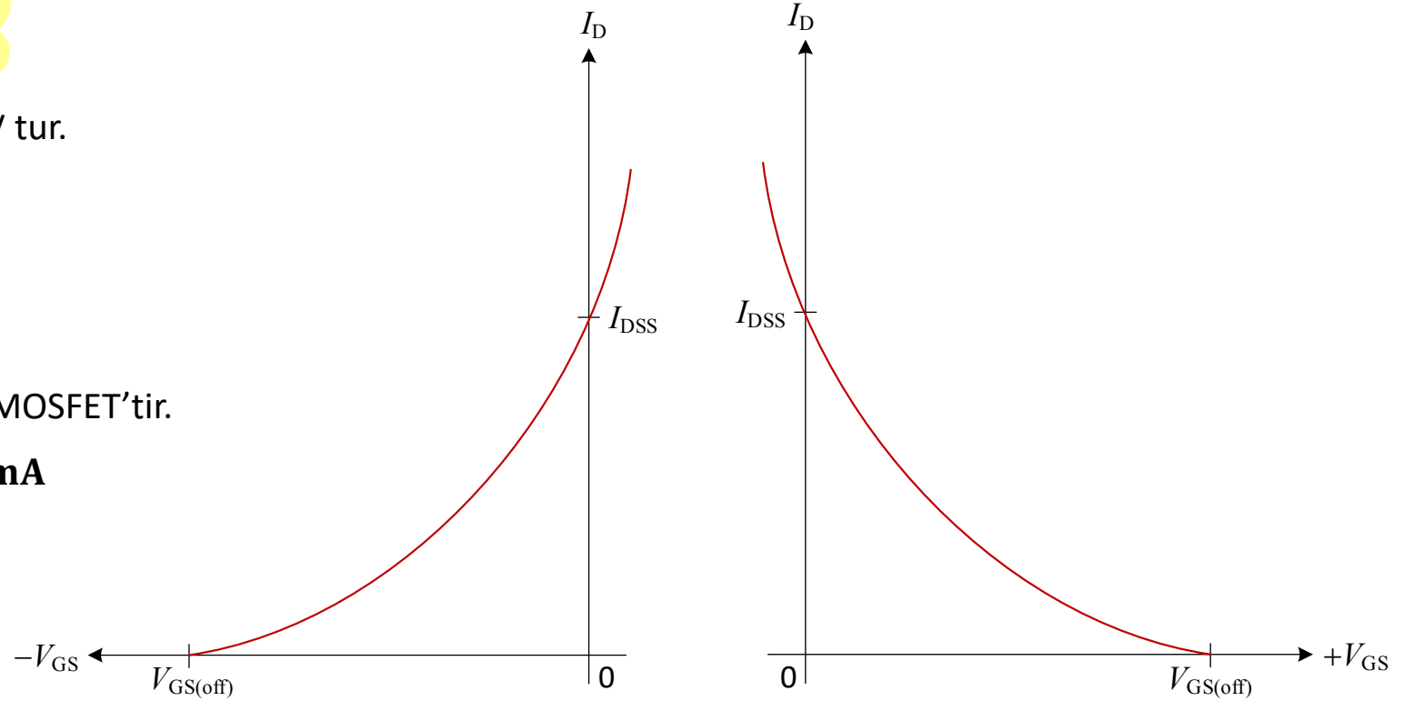
Şekil 16 (a) n -kanal
