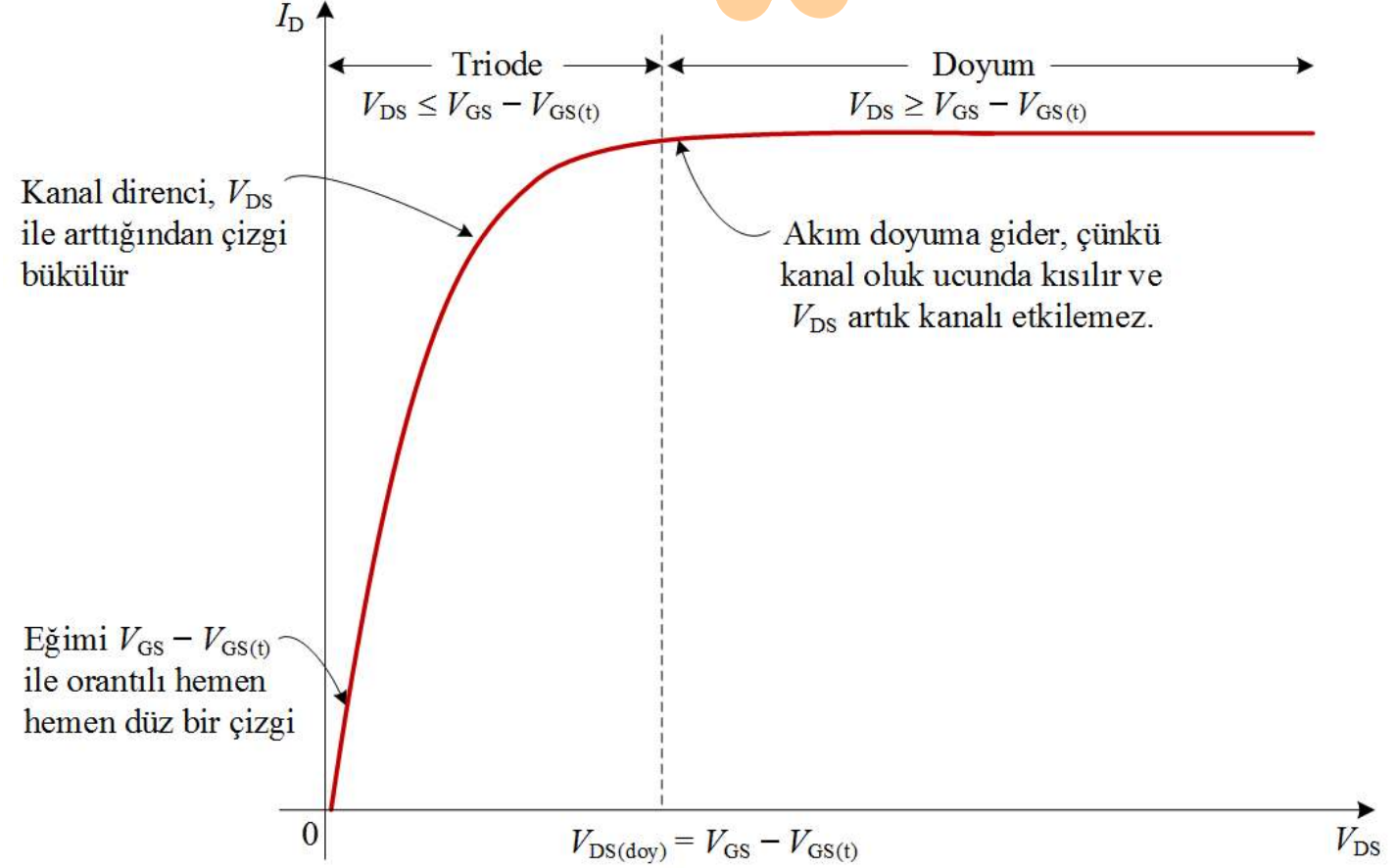
(b) V_{GS} - V_{GS(t)} ile çalışan bir n-kanal üretim tipi MOSFET için oluk-kaynak voltajı V_{DS} ye karşı oluk akımı I_D nin değışimi.
